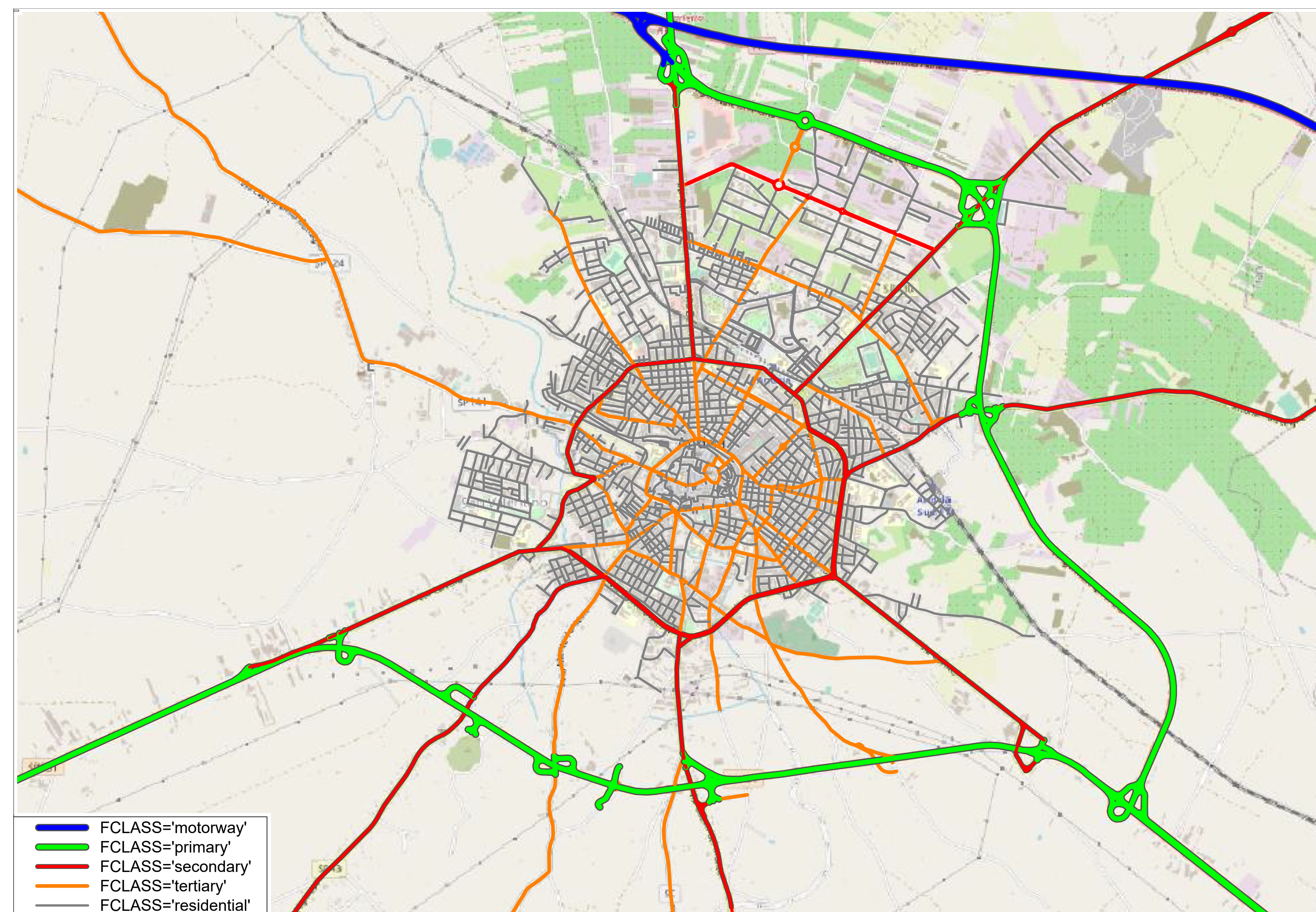
Scenario Attuale - rappresentazione grafo stradale classificato
