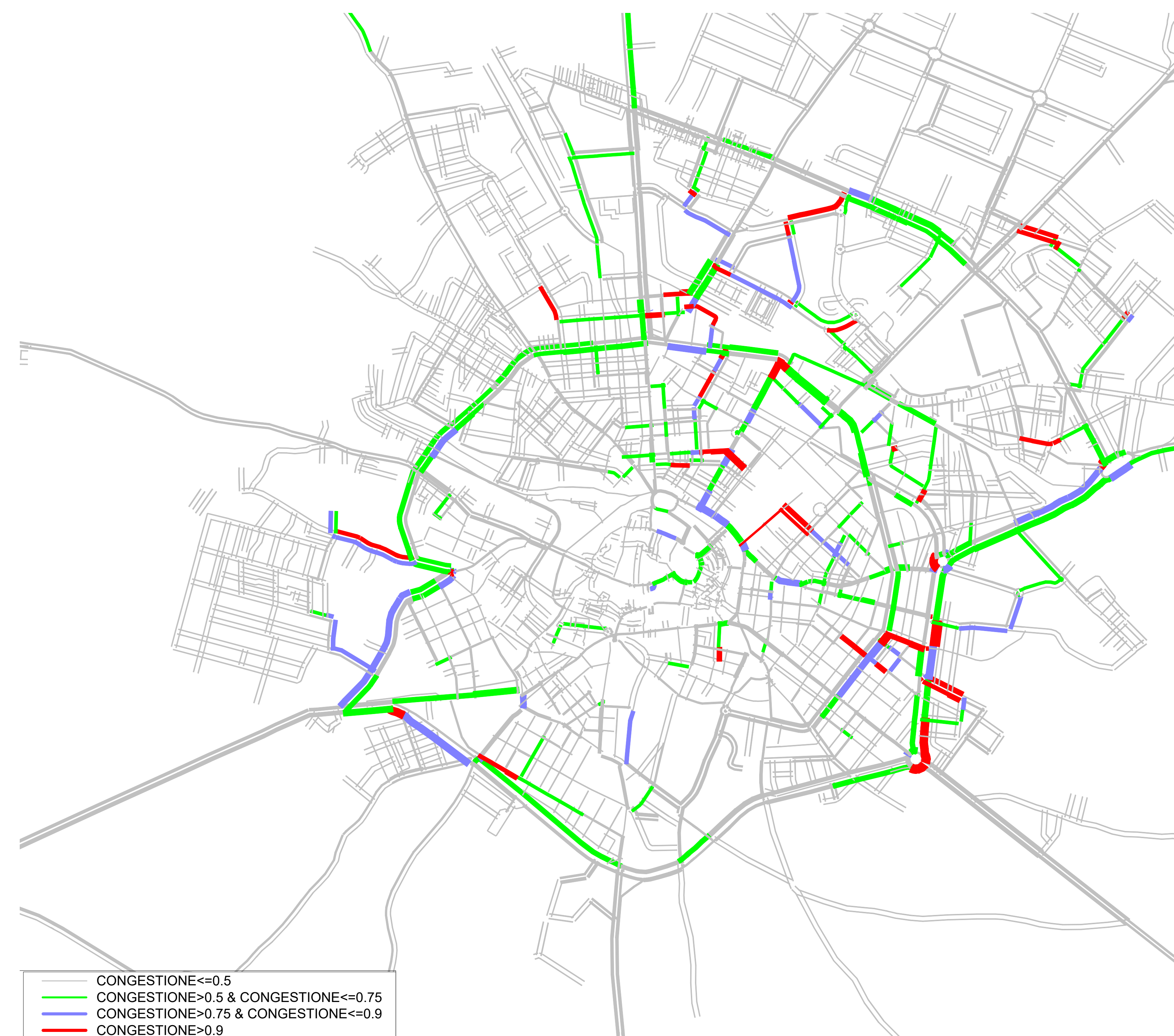
Scenario Futuro - congestione (flusso/capacità) ora di punta del mattino (8-9)
