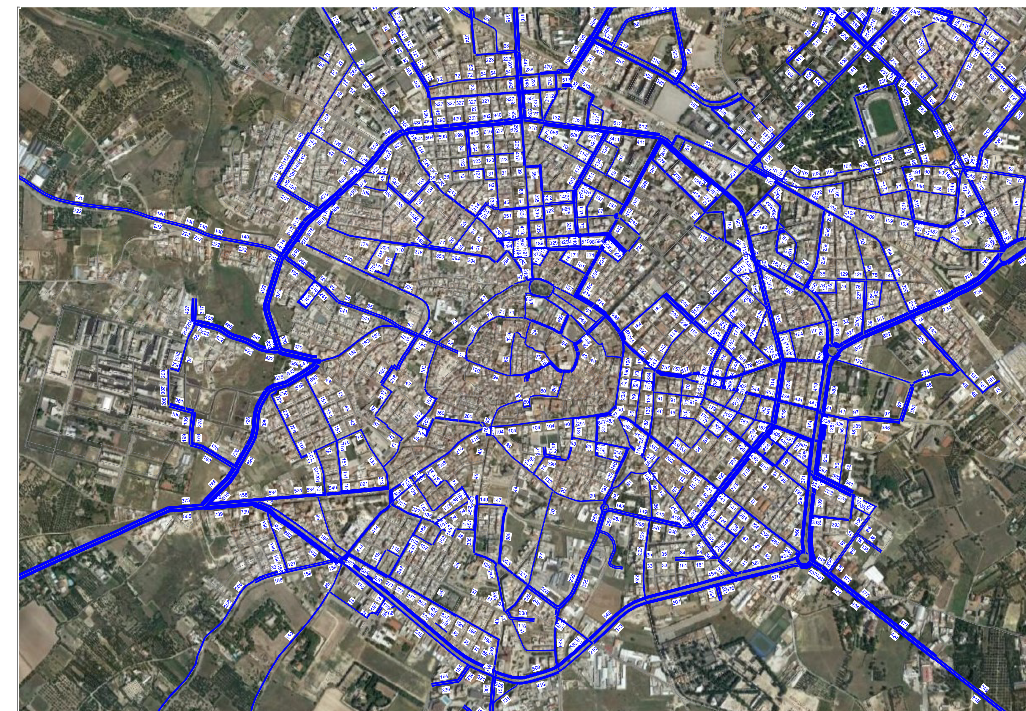
Scenario Futuro - flussogramma ora di punta del mattino (8-9) in veicoli equivalenti
